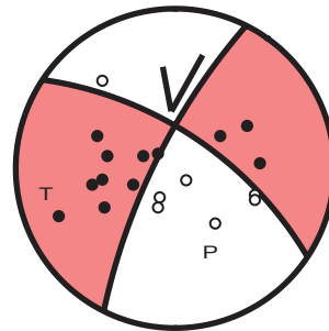
23/04/2017 17h 47mn 17s ML = 2.6 ( 207, 76, -27 )
